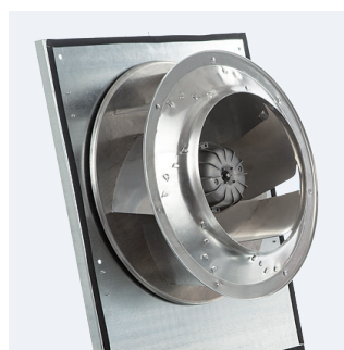
Dynamicznie wyważony wirnik z łopatkami pochylonymi do tyłu
